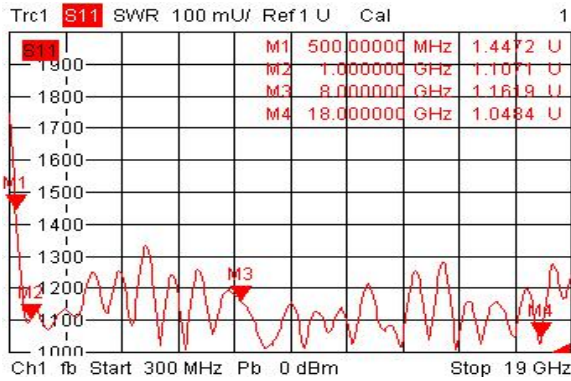
1.输入驻波比 Input VSWR
