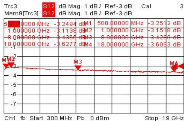
5.损耗及幅度平衡 Loss&Amplitude Unbalance
