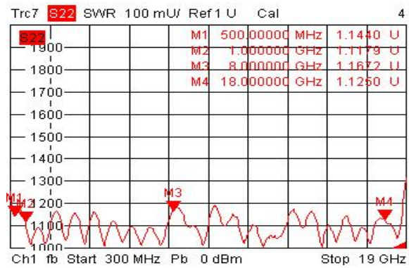
2.输出驻波比 Output VSWR
